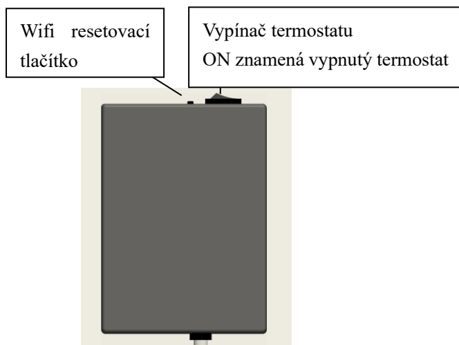
Přijímač na zadní části panelu
